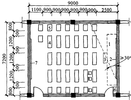
附图3 中学普通教室平面布置示意图
