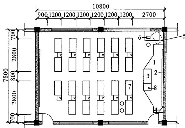
附图2 小学科学教室平面布置示意图
