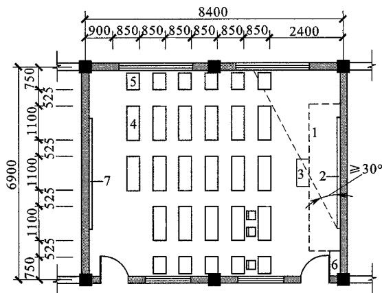
附图1 小学普通教室平面布置示意图
