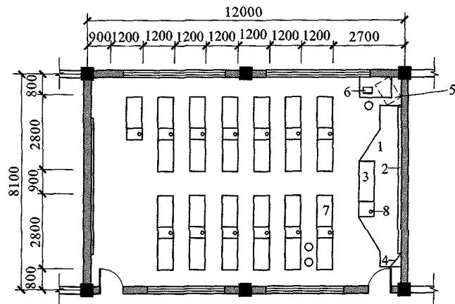
附图4 中学化学、生物实验室平面布置示意图
